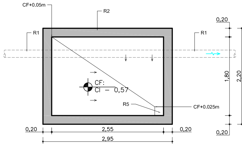
PLANTA Nivel: 1-1
