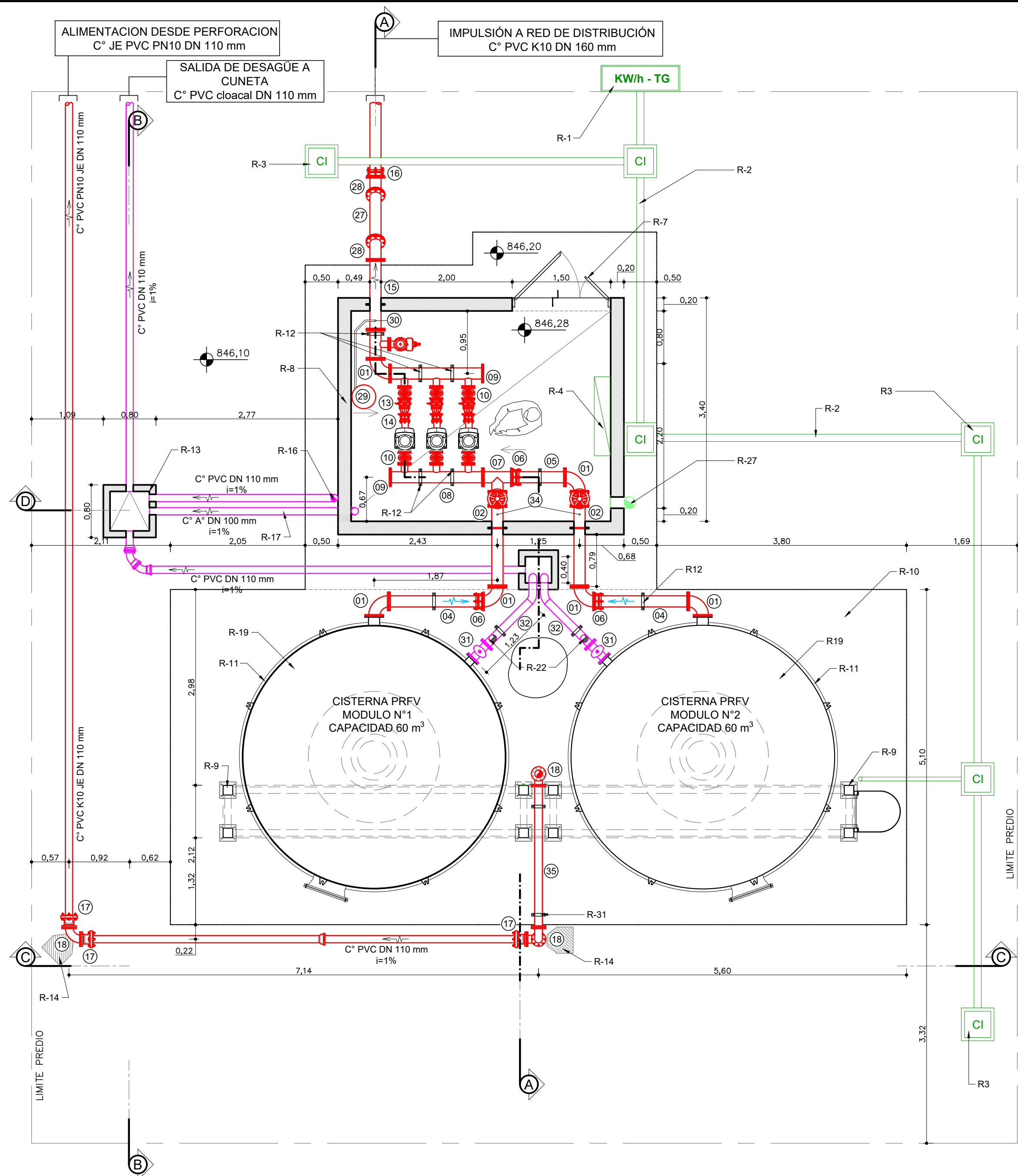
PLANTA - Nivel 1-1
