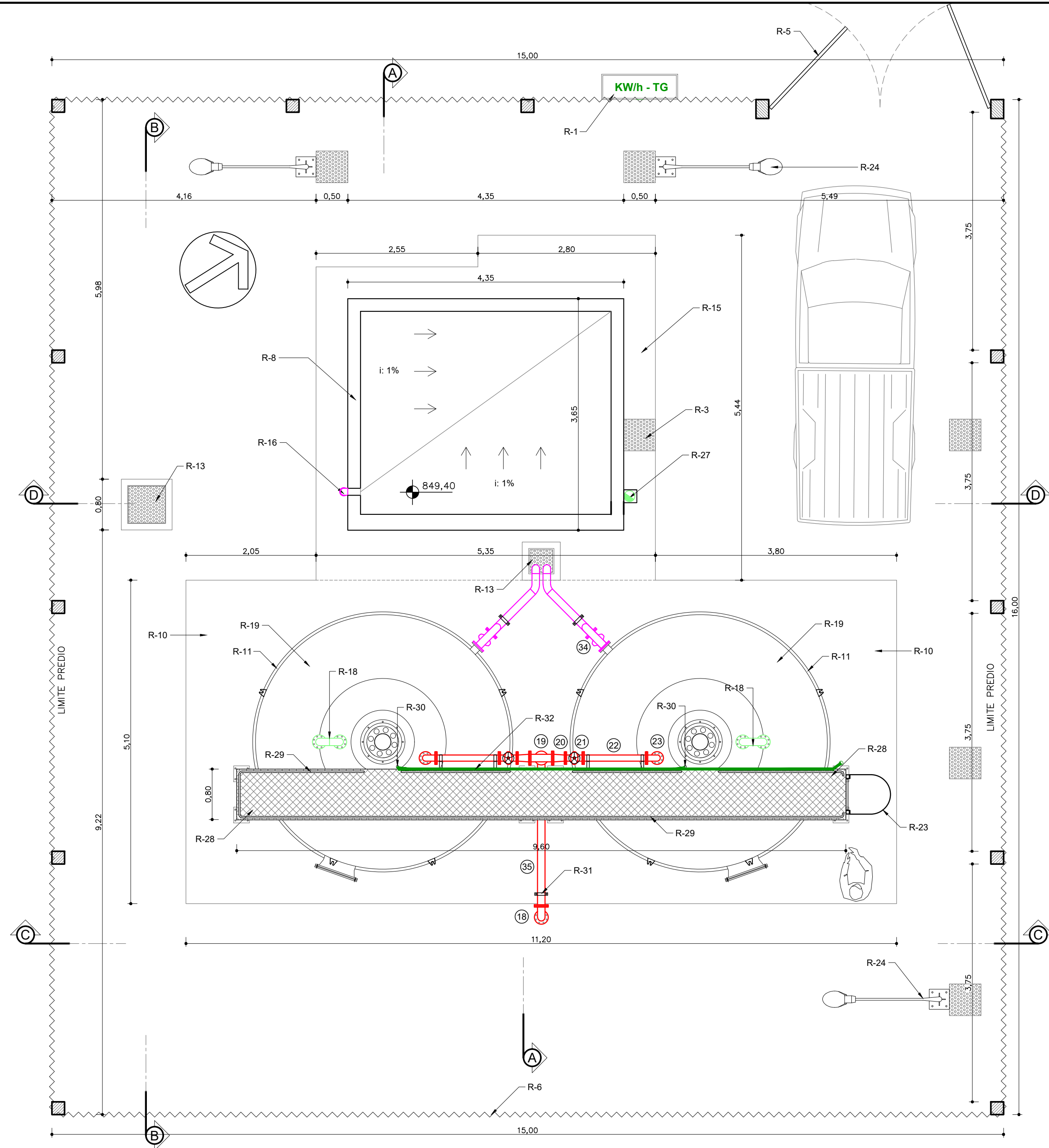
PLANTA - Nivel 3-3
