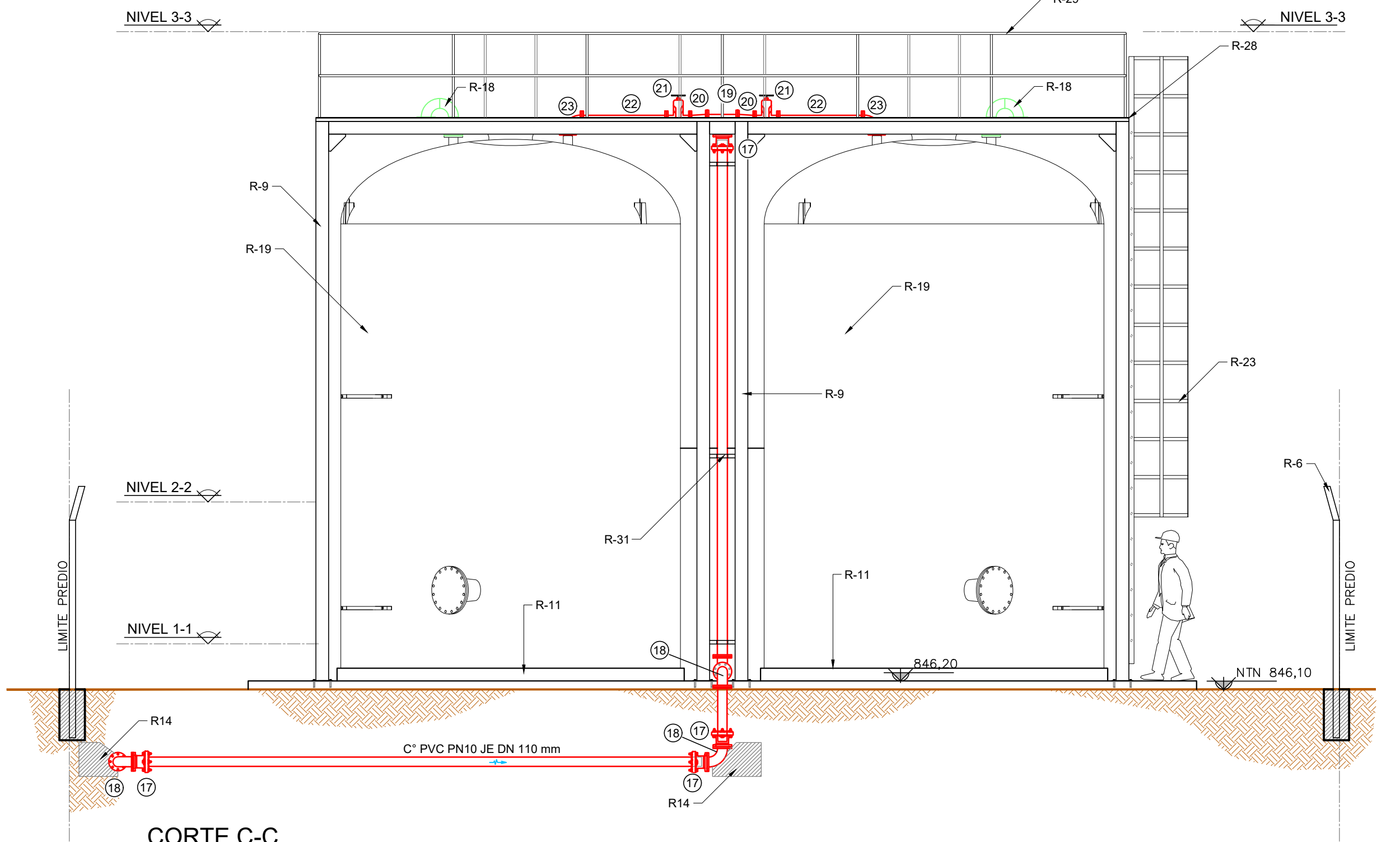
CORTE C-C
