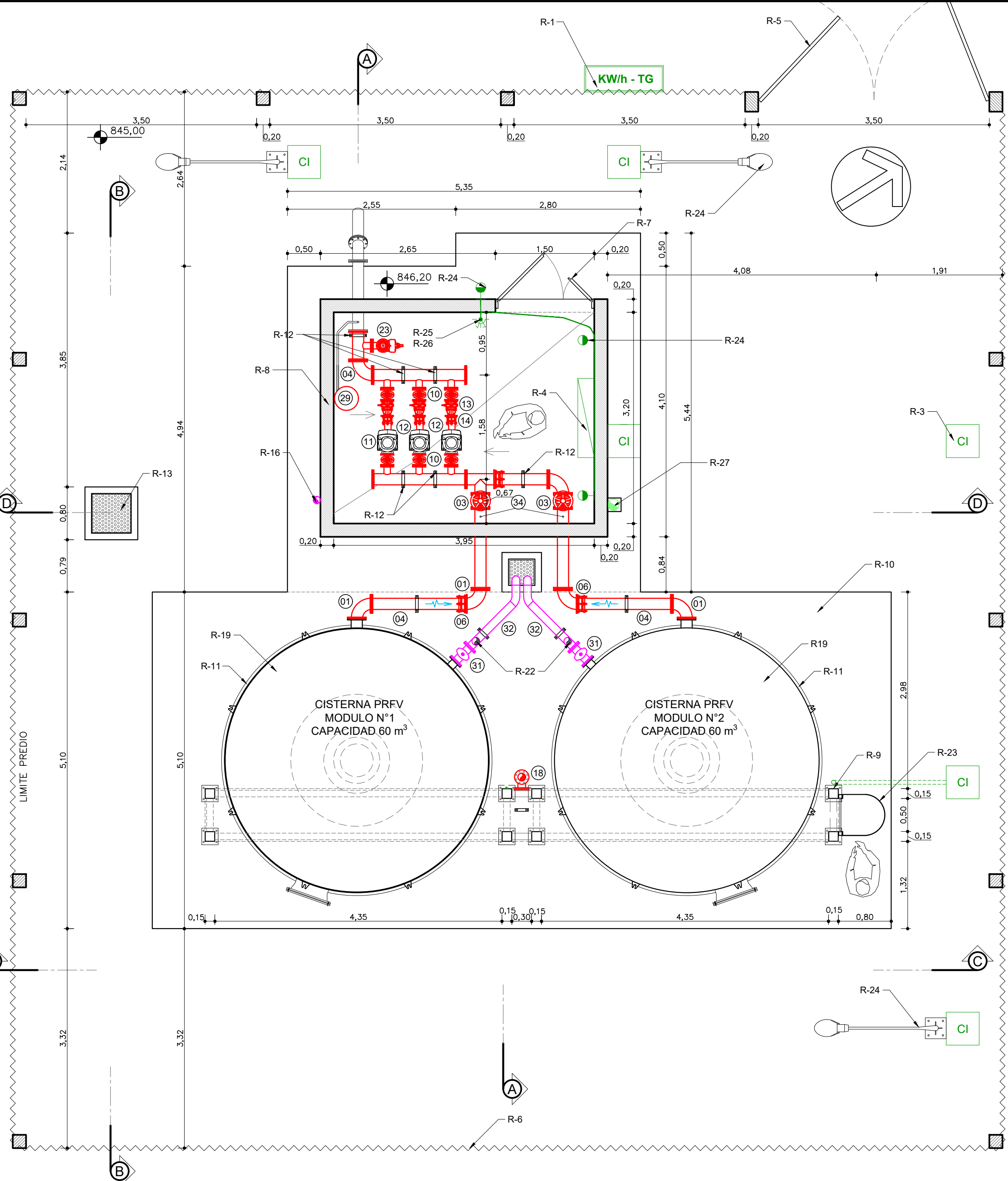
PLANTA - Nivel 2-2
